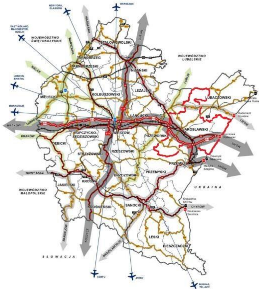
Mapa 18 Zewnętrzna dostępność komunikacyjna województwa podkarpackiego
